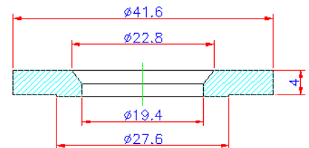
Borracha da Enchedora DLDB 408S
