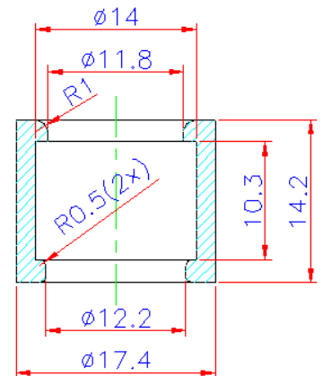
Borracha da Enchedora DLDB 408S
