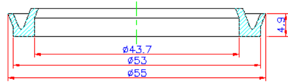
Gaxeta GDI 675 - DLDB 5613950
