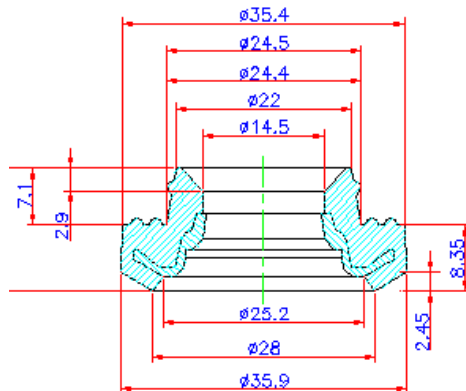
Retentor do Barril Keg DLDB 3518
