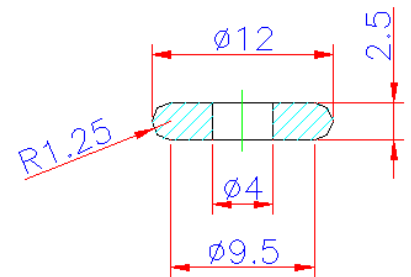
Vedação da Agulha Maior GEA863 DLDB 5161657
