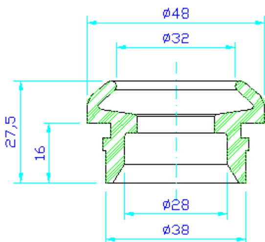
Borracha de Vedação 133331
