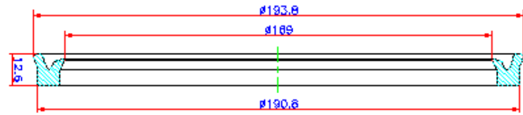
Gaxeta GDI 675 - DLDB 5613950
