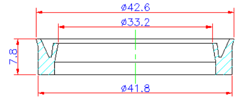
Gaxeta GAD 141 - DLDB 1061266
