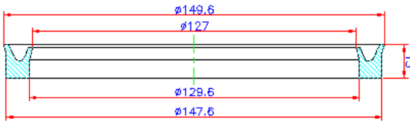
Gaxeta GTI 500 - DLDB 5160995
